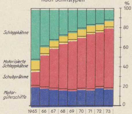
Transportmenge der Binnenschifffahrt nach Schiffstypen
